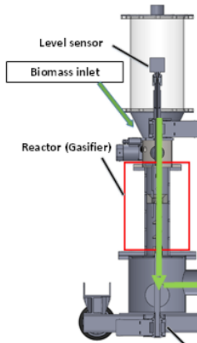
Gambar 5. Penampang Downdraft Gasifier Pada Experiment
