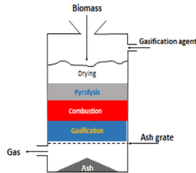
Gambar 2. Penampang Downdraft Gasifier secara umum
