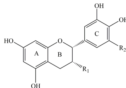
Fig. 1. Catechin molecule
