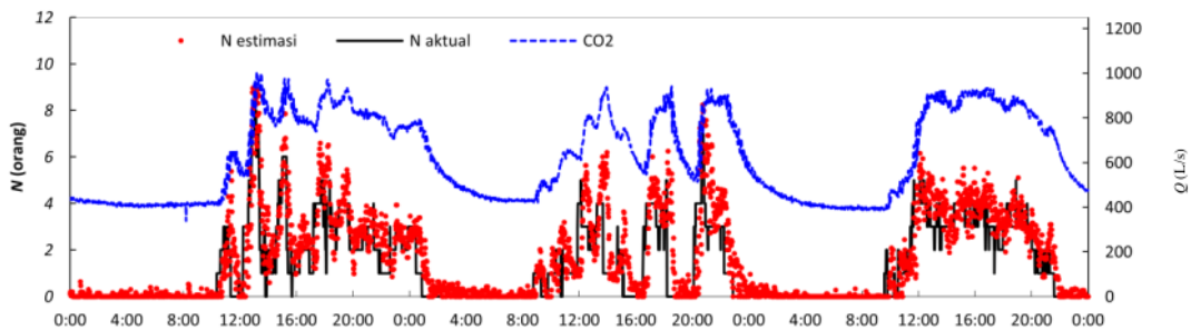
Gambar 2. Profil \text{CO}_2 , jumlah penghuni aktual dan estimasi pada skema kontrol ventilasi kedua
