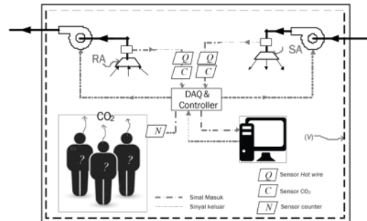
Gambar 1. Layout sistem kontrol
