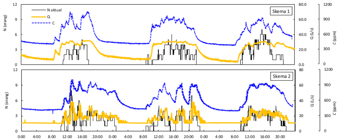
Gambar 5. Profil laju ventilasi pada skema 1 dan 2
