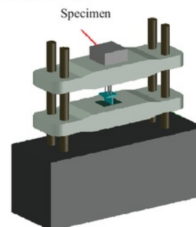
Fig. 1 Pullout Test
